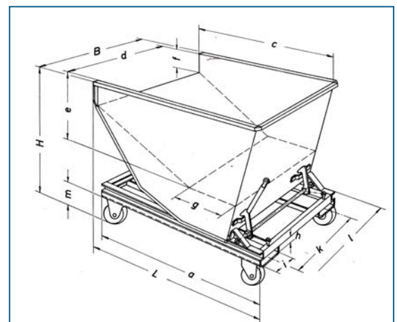
Ausführung für Hebelrollereinsatz
