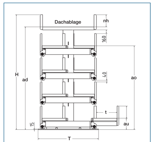
Ausführung doppelseitig
